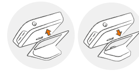
Befestigen des Ständers B.Box Evo oder des Akkuhalters B.Box Evo
